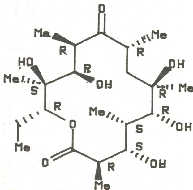
ERYTHRONOLIDE A
